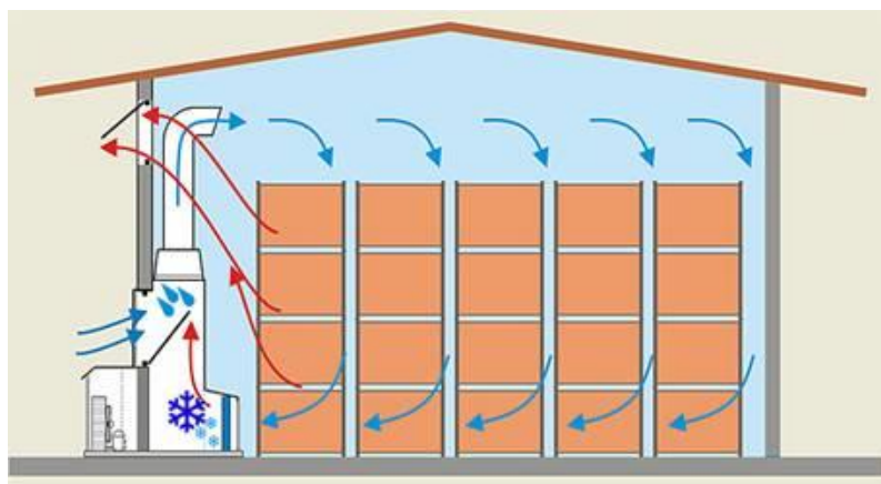
Схема системы вентиляции хранилищ построенной на базе Агробизнес - центра
